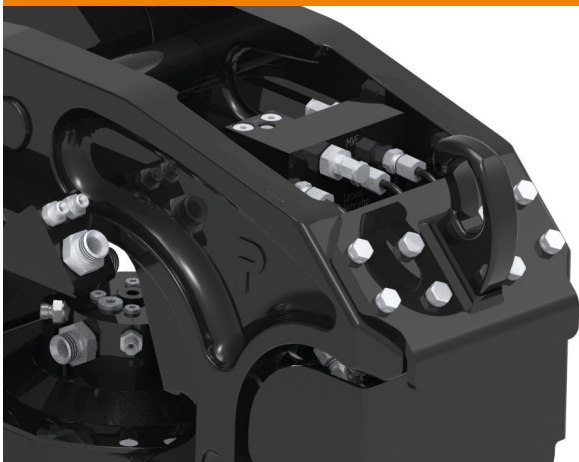
Crochet de charge pour 3 tonnes
