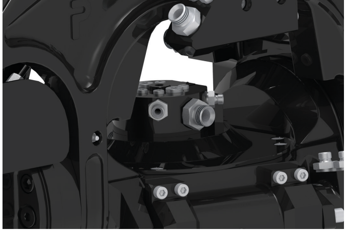
Large transmission de pivotement à 7 canaux
