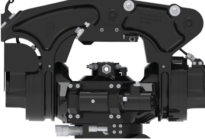
Concept de pivotement innovant avec moteur à pistons radiaux
